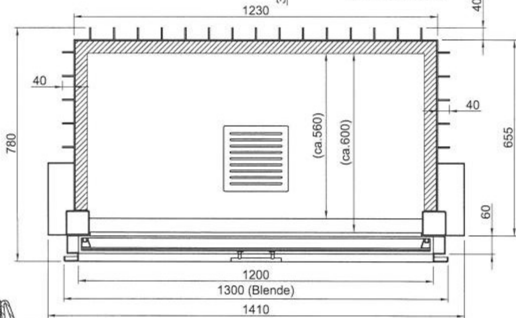
Geschlossenes Türprofil, ohne Anpresstechnik
